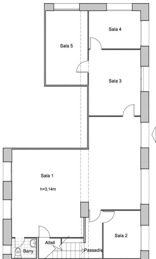
PLANTA BAIXA
