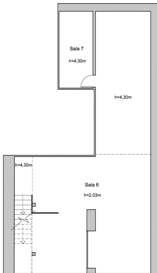
PLANTA SOTERRÀNIA
